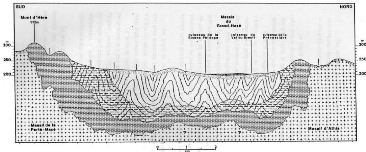
fig. 4 : COUPE GÉOLOGIQUE SCHEMATIQUE
